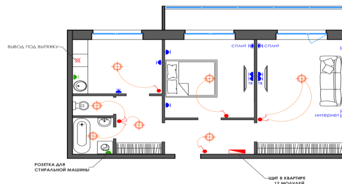
ПЛАН ЭЛЕКТРИКИ 2Х КОМНАТНОЙ КВАРТИРЫ
