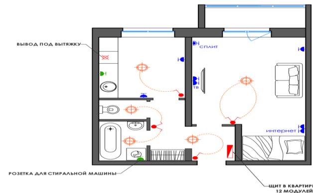
ПЛАН ЭЛЕКТРИКИ 1 КОМНАТНОЙ КВАРТИРЫ
